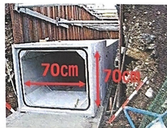
水路据付状況
